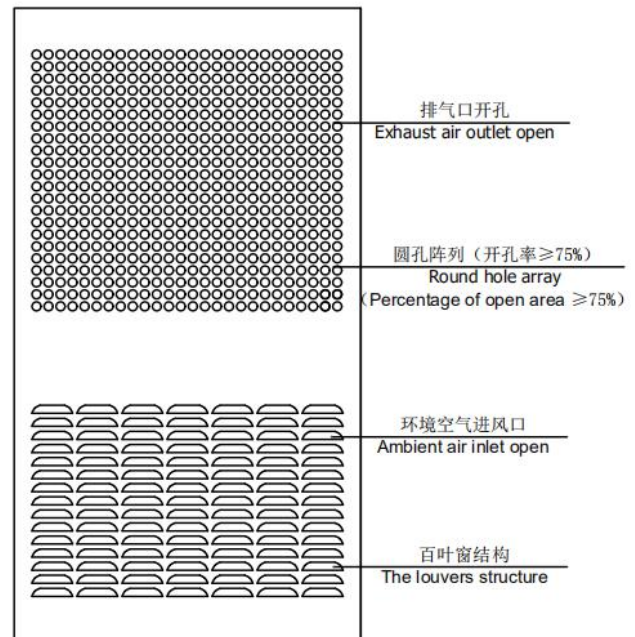
图 3-安装示意图
