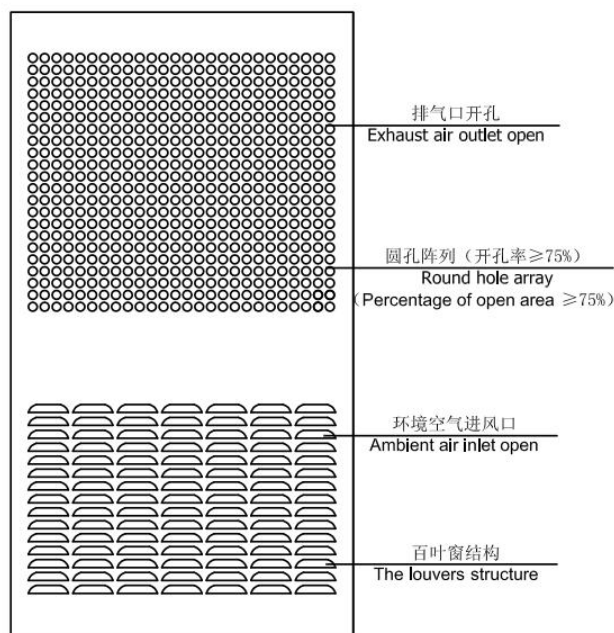
图 3-安装示意图
